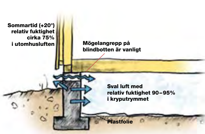
”Modern” kryppgrund, uteluftsventilerad.
