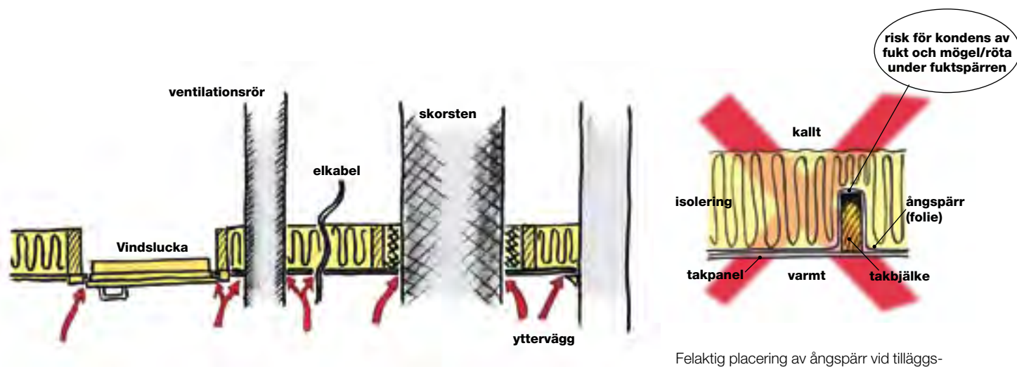
Riskställen för fuktig varmluft att tränga upp i vindsutrymmet.
