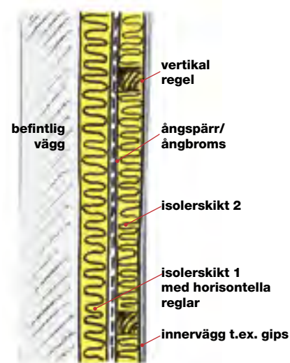
Exempel på utförande av invändig isolering av yttervägg sett uppifrån.
